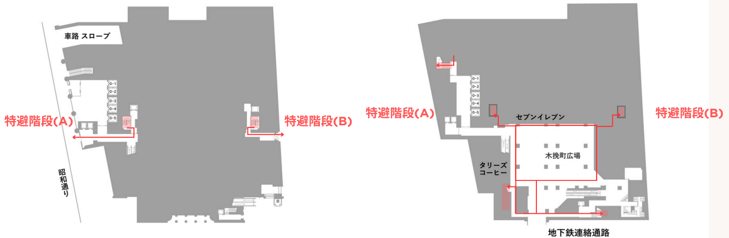
避難階（1F）
